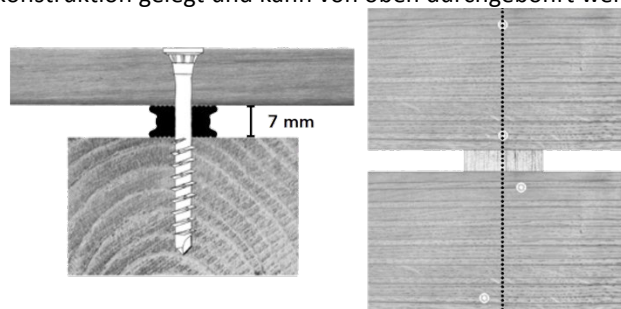
Terrassenaufbau mit Distanzprofil und Schraubenanordnung in Linie bzw. versetzter Anordnung
